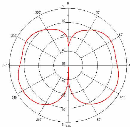
AN0835 E-Plane
