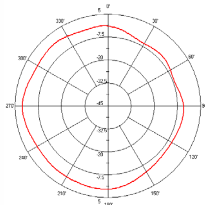
AN0835 E-Plane
