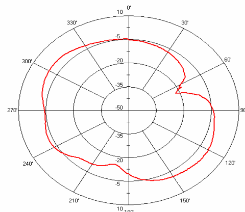
AN6520 E-Plane
