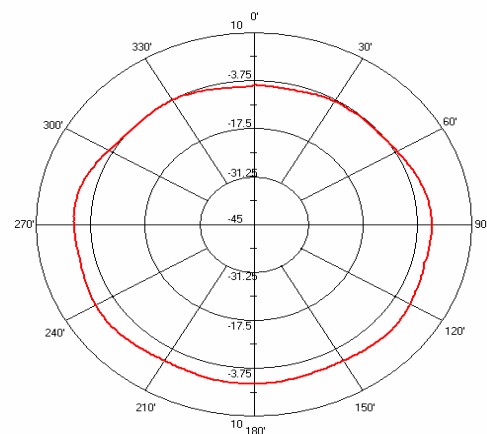
AN6520 E-Plane
