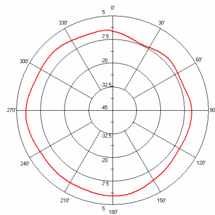
AN7638 E-Plane
