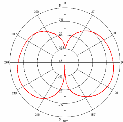
AN7638 E-Plane
