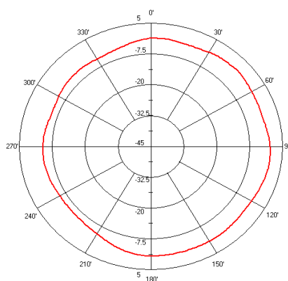
AN2051 E-Plane
