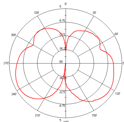
AN2051 E-Plane
