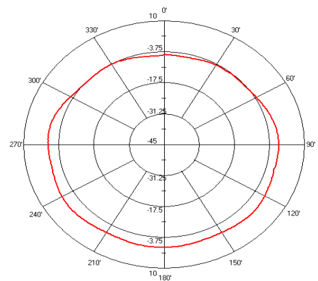
AN6520 E-Plane
