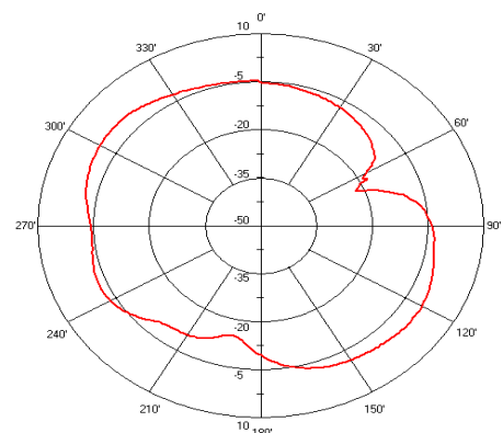
AN6520 E-Plane
